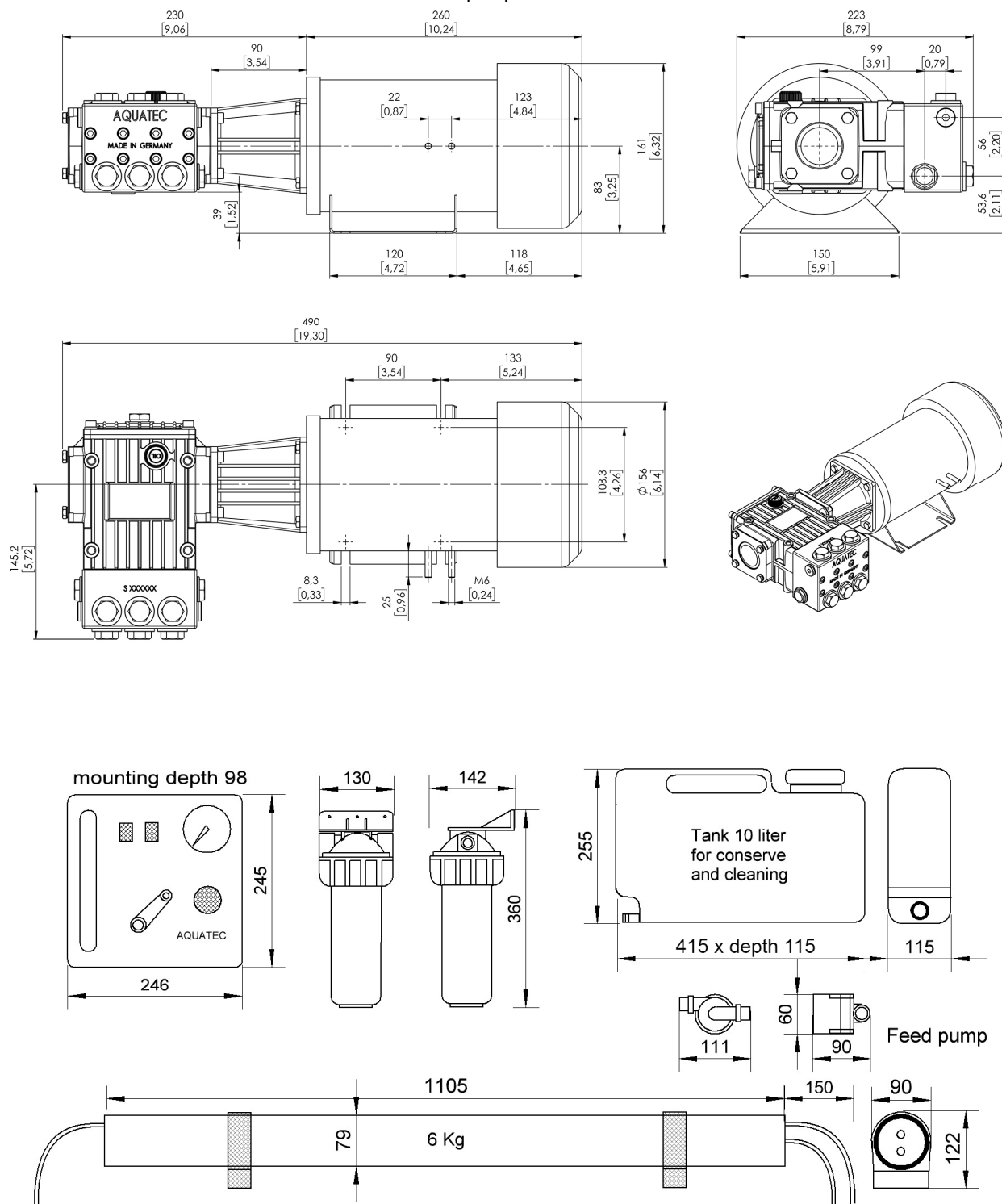
Motor pump unit DD 500
